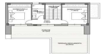
PLANTA PRIMERA
